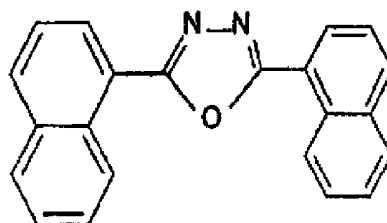
BND
