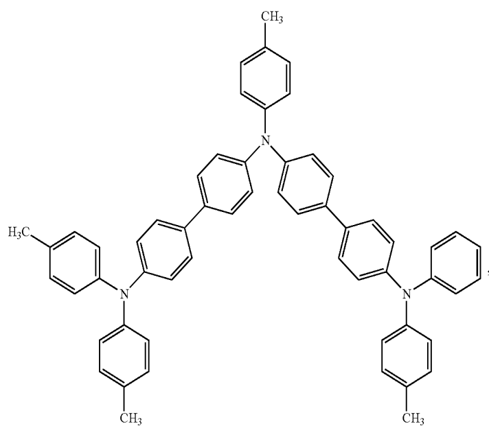
HTM-1
