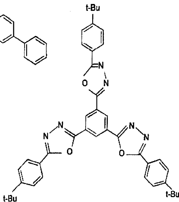
OXD-Star
