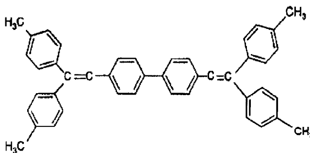
DTVb1
