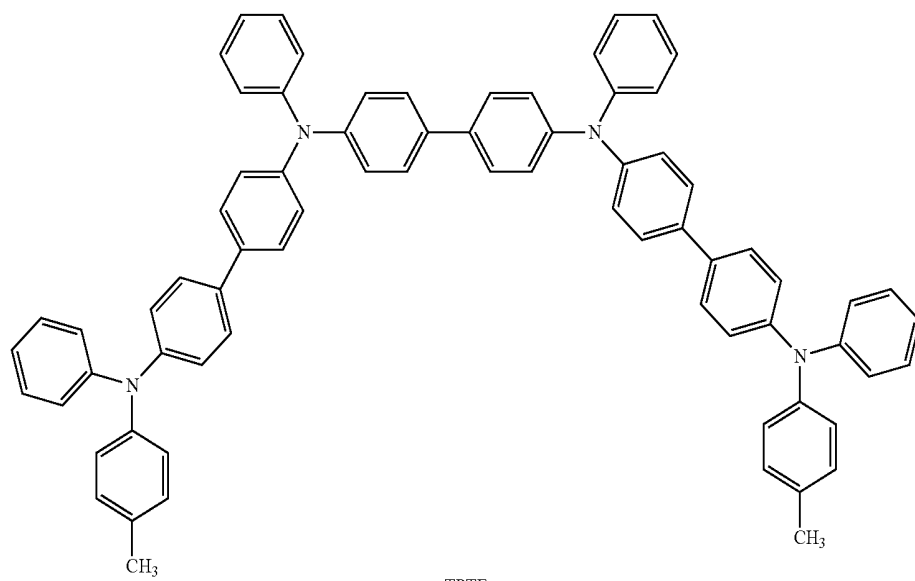
TPTE
