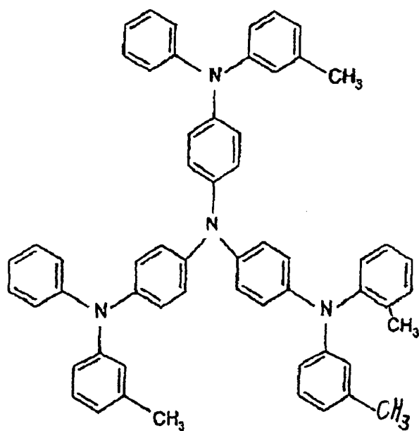
mTADATA
