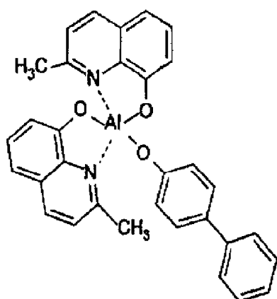
BAlq1
