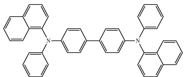
\alpha -NPS
