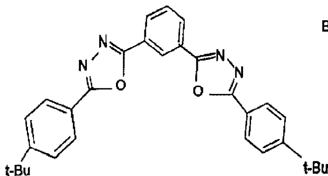
OXD-7
