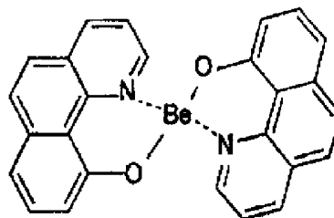
Bebq
