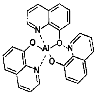
Alq
